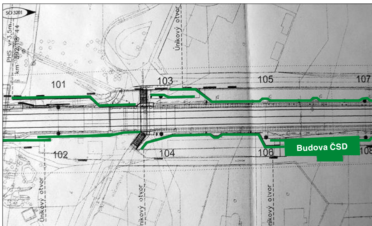
Obr. 2. - Návrh rozmístění protihlukových stěn v prostoru železniční stanice
