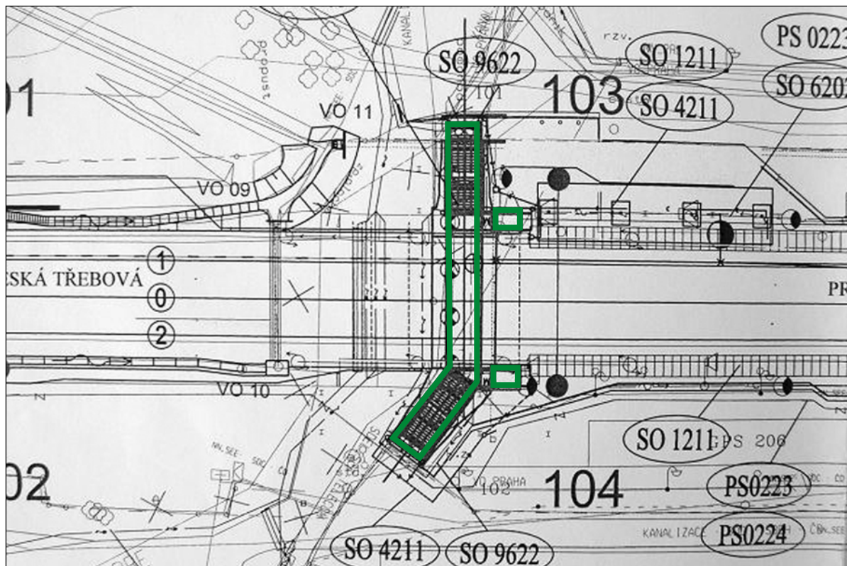
Obr. 1. - Schéma podchodu s umístěním 2 bezbariérových výťahů
