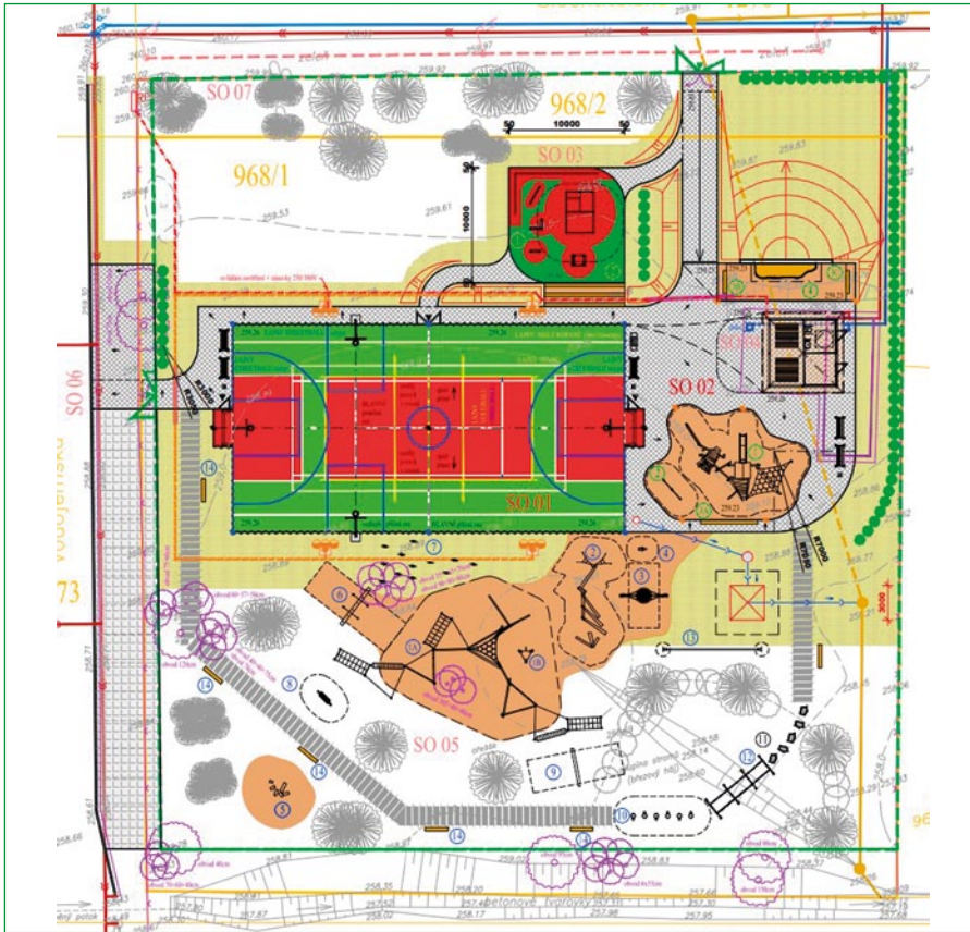
Celková situace projektu hřiště na „Kavrisu“ včetně druhé etapy Výkres: Jan Dudr PROJEKTOVÁNÍ SPORTOVIŠTĚ
