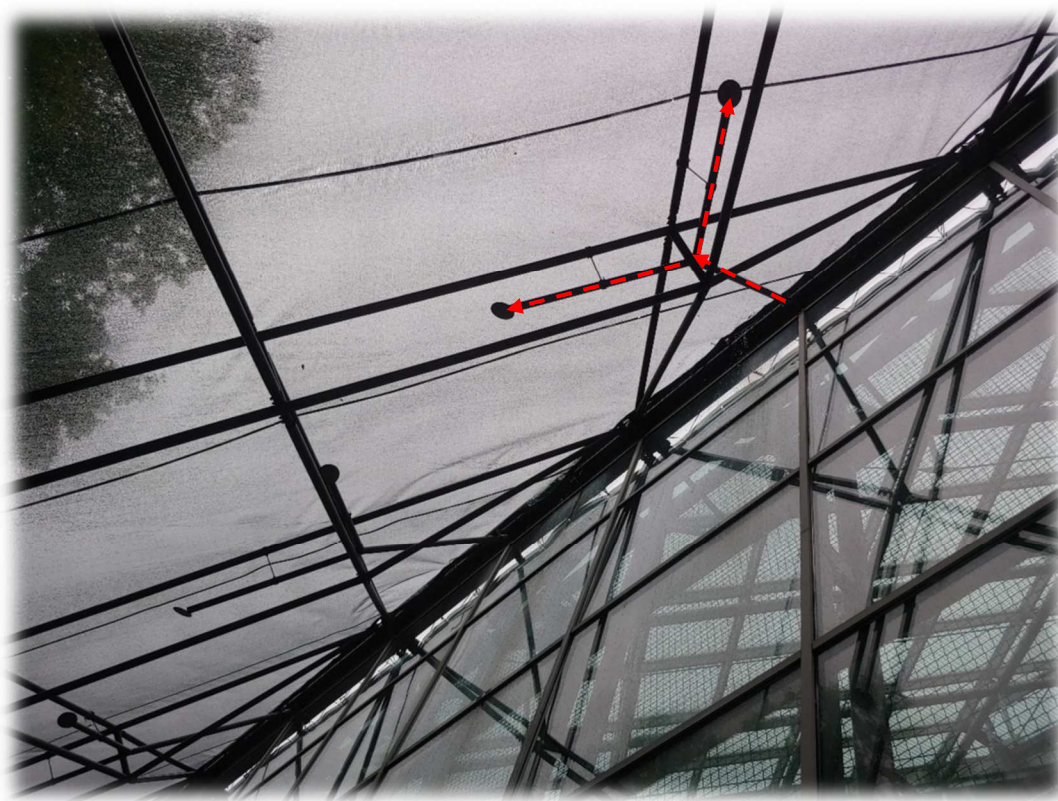
Obrázek 17: Sportovní hala starosty Hanzela – nevhodné řešení dešťových svodů
