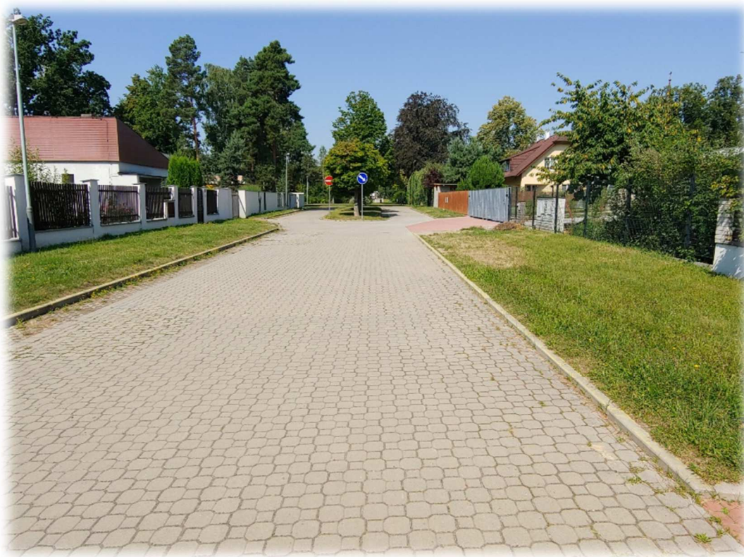
Obrázek 30: Ul. Utěšilova – po levé straně vsakovací pás z betonových zatravnovacích prvků, lepšímu vsakování zabraňuje zvýšený obrubník po obou stranách komunikace (nedostatky)
